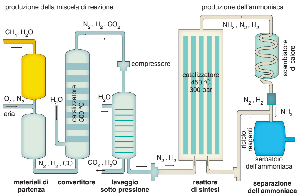
◀ Figura 1 Rappresentazione schematica di un impianto industriale per la produzione di ammoniaca. In questo schema compaiono anche le fasi di preparazione dei reagenti.
